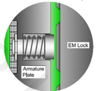
EM Lock De-energized
